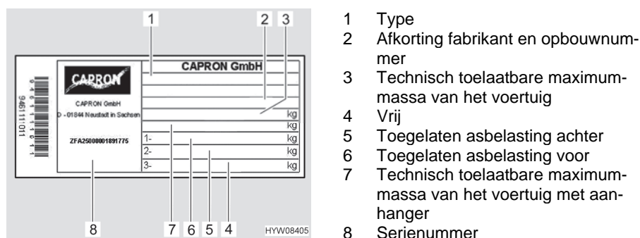
Afb. 125 Typeplaatje
