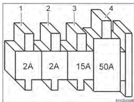
Afb. 83 Zekeringen op de startaccu
