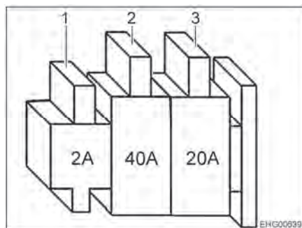
Afb. 85 Zekeringen bij één woonruimteaccu
