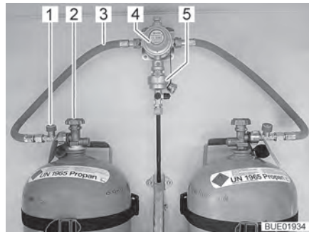
Afb. 67 Gasflessen met DuoControl
