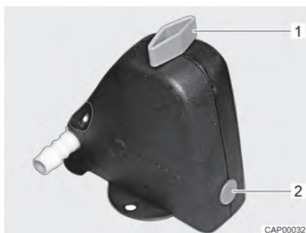
Afb. 109 Veiligheids-/aftapventiel gesloten
