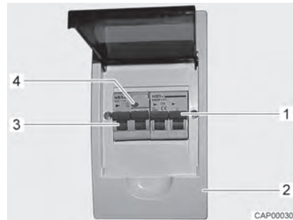
Afb. 78 Beveiligingsautomaat en FI-schakelaar (230-V-zekeringenkast)
