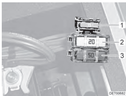
Afb. 81 Zekeringen op de startaccu zonder laadbooster
