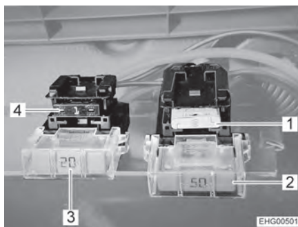
Afb. 84 Zekeringen op de woonruimteaccu met laadbooster
