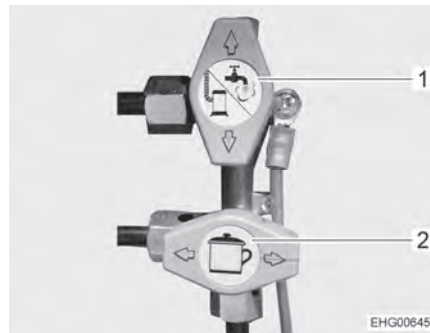
Afb. 73 Gasafsluitkranen
