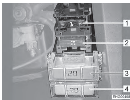
Afb. 82 Zekeringen op de startaccu met laadbooster
