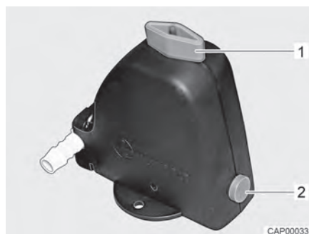
Afb. 105 Veiligheids-/aftapventiel geopend
