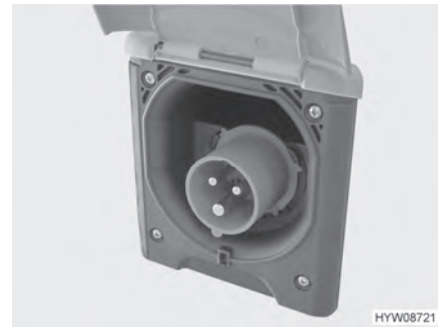
Afb. 79 230-V-aansluiting op het voertuig (CEE-contactdoos)
