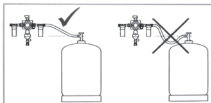
Afb. 71 Correcte aansluiting van de gasfles
