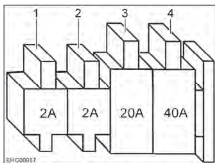
Afb. 86 Zekeringen bij twee woonruimteaccu's
