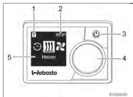
Afb. 95 Bedieningspaneel (standverwarming)
